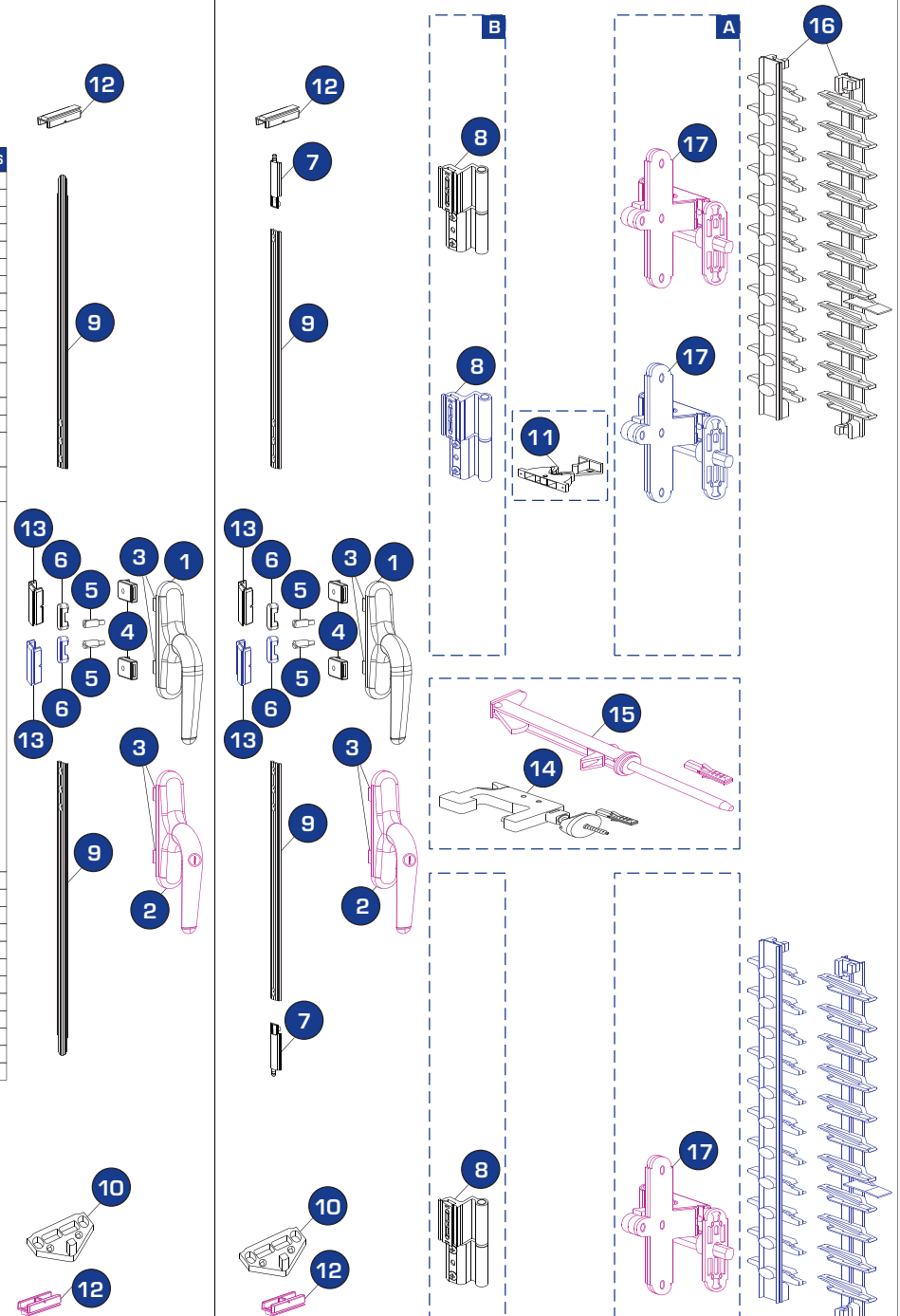
Μηχανισμός τετράφυλλου παντζουριού -πρώτα φύλλα-
