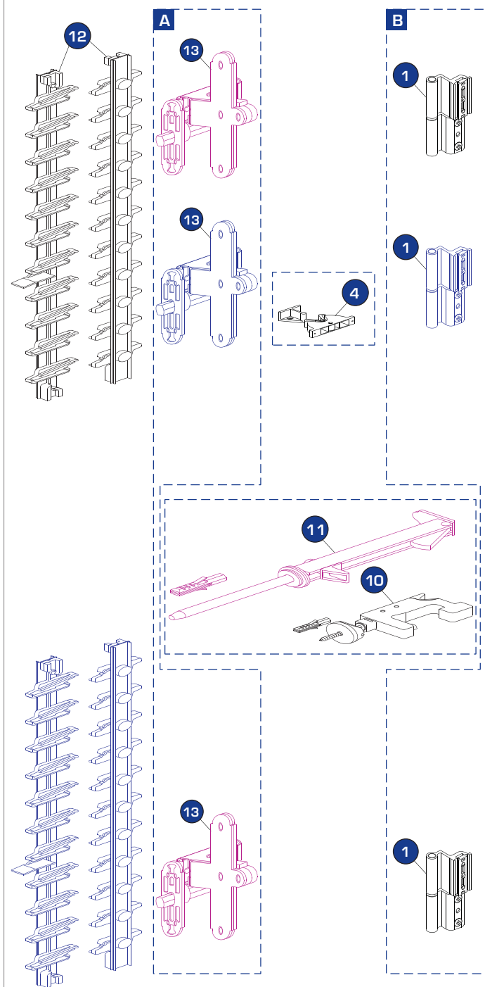
Μηχανισμός τετράφυλλου παντζουριού -δεύτερα φύλλα-
