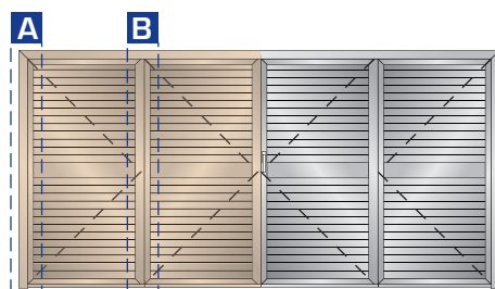
Μηχανισμός τετράφυλλου παντζουριού -δεύτερα φύλλα-
