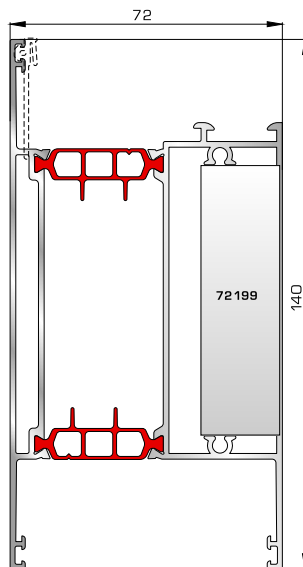
Ταμπλάς φύλλου (για φύλλα 80875, 80895)
