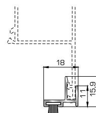
Προφίλ επικάλυψης (για ταμπλάδες 81325, 81355)
