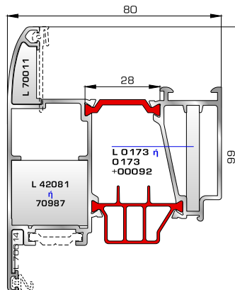
Φύλλο πόρτας εισόδου ανοιγόμενης έξω
