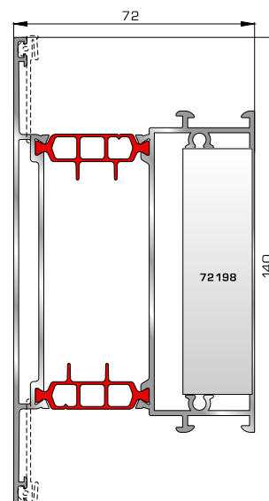
Μεγάλο ταφ φύλλου (για φύλλα 80365, 80315, 80895, 80875)
