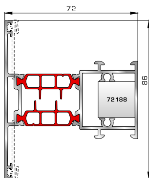
Ταφ φύλλου (για φύλλα 80365, 80315, 80895, 80875)
