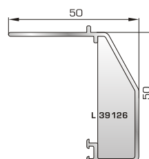
39125 W=493gr/m A=0,248m 2 /m Αρμοκάλυπτρο σπαστό βιδωτό 50mm
