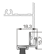
42795 W=158gr/m A=0,097m 2 /m Προφίλ επικάλυψης (για ταμπλάδες 50775, 50555)
