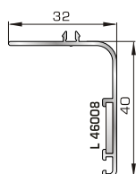
46125 W=271gr/m A=0,176m 2 /m Αρμοκάλυπτρο επίπεδο βιδωτό 40mm
