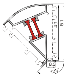
50415 W=791gr/m A=0,229m 2 /m Προφίλ γωνιακής σύνδεσης 135°
