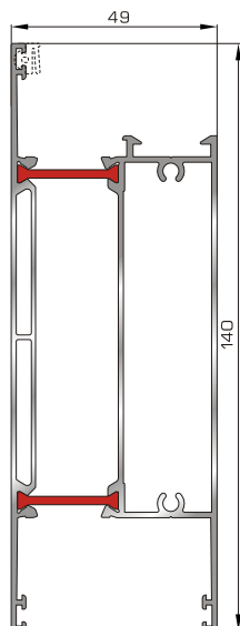
50555 W=2035gr/m A=0,522m 2 /m Ταμπλάς φύλλου 49mm (για φύλλα 50108, 50204)
