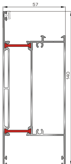
50775 W=2090gr/m A=0,542m 2 /m Ταμπλάς φύλλου 57mm (για φύλλα 50865, 50203)
