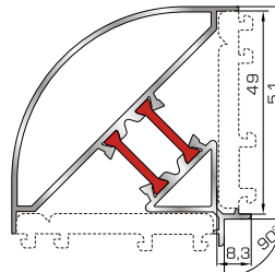
50435 W=1101gr/m A=0,284m 2 /m Προφίλ γωνιακής σύνδεσης 90°
