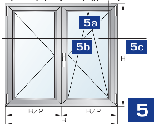
Δίφυλλο ανοιγο-ανακλινόμενο με περιμετρικό μηχανισμό
