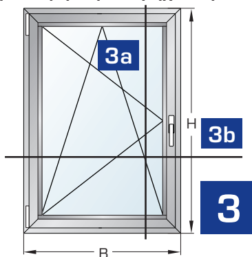
Μονόφυλλο ανοιγο-ανακλινόμενο με περιμετρικό μηχανισμό
