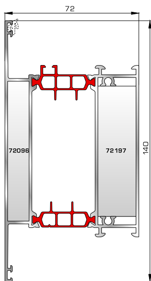
Μεγάλο ταφ κάσας
