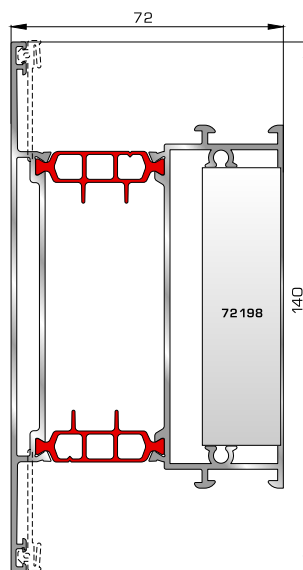
Μεγάλο ταφ φύλλου (για φύλλα 80895, 80875)
