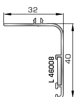
Αρμοκάλυπτρο επίπεδο βιδωτό 40mm
