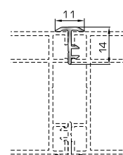
Αρμοκάλυπτρο κουμπωτό ένωσης δυο κασών
