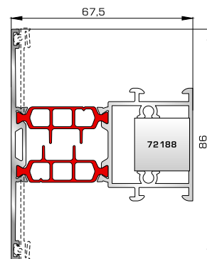
Ταφ φύλλου 67,5mm (για φύλλα 80915, 80965)
