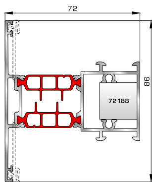
Ταφ φύλλου 72mm (για φύλλα 80895, 80875)
