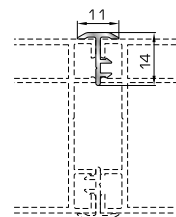
Αρμoκάλυπτρο κουμπωτό ένωσης δύο κασών
