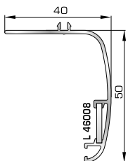
Αρμoκάλυπτρο πομπέ βιδωτό 50mm
