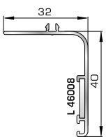
Αρμoκάλυπτρο επίπεδο βιδωτό 40mm
