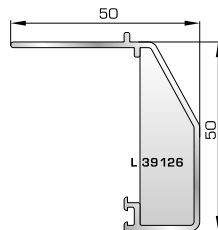
Αρμoκάλυπτρο σπαστό βιδωτό 50mm
