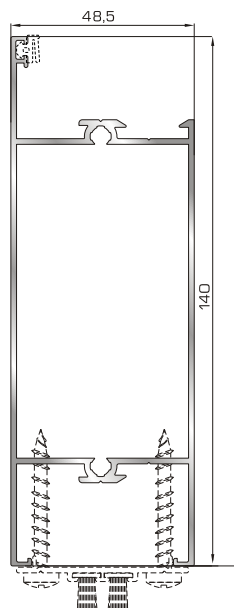
Ταμπλάς φύλλου
