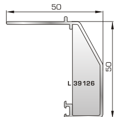
Αρμοκάλυπτρο σπαστό βιδωτό 50mm
