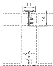
Αρμοκάλυπτρο κουμπωτό ένωσης δύο κασών
