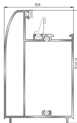
Ταμπλάς κάσας Rondo
