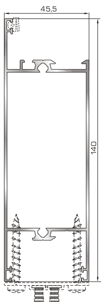
Ταμπλάς κάσας
